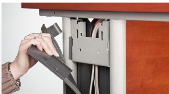
Ukrytí kabeláže – detail jednoduchého a originálního vedení kabelů vnitřkem nohy
